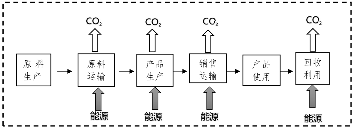
图 2 平型钢材树脂砂轮产品生命周期评价边界图
