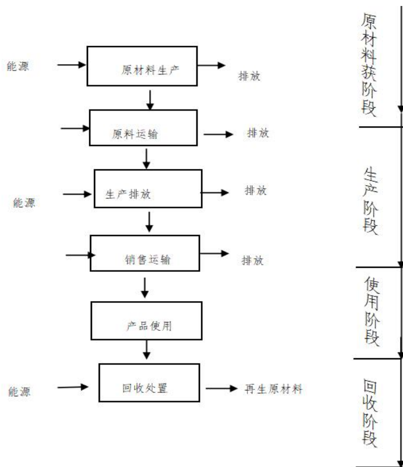
图 1 平型钢材树脂砂轮生命周期系统边界图
